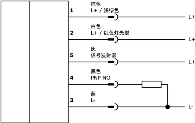
连接图 EZ550320
