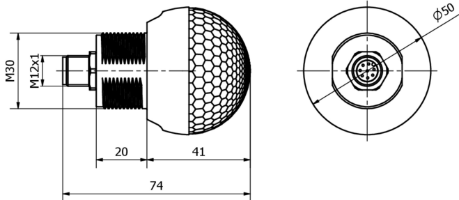
尺寸图 EZ360330
