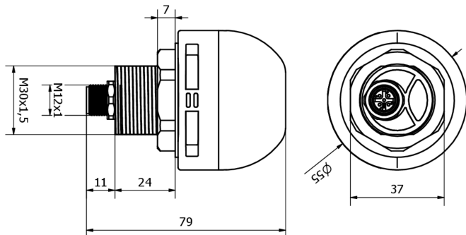
尺寸图 EZ550320
