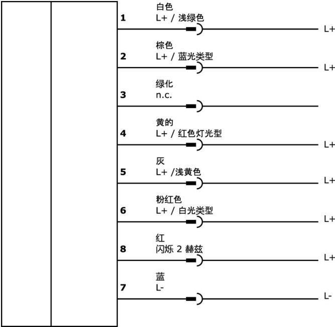
连接图 EZ550320
