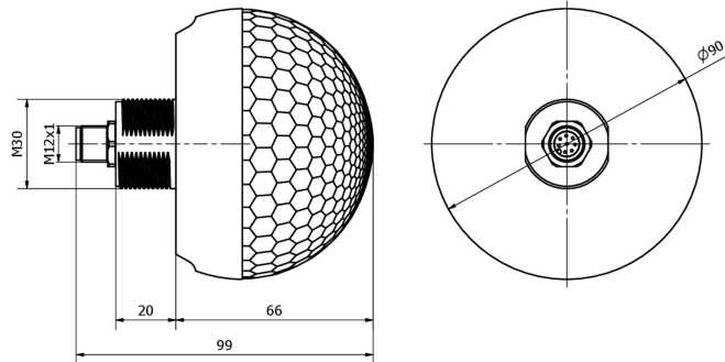
尺寸图 EZ360331
