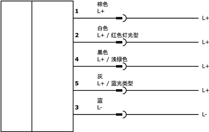
连接图 EZ650520
